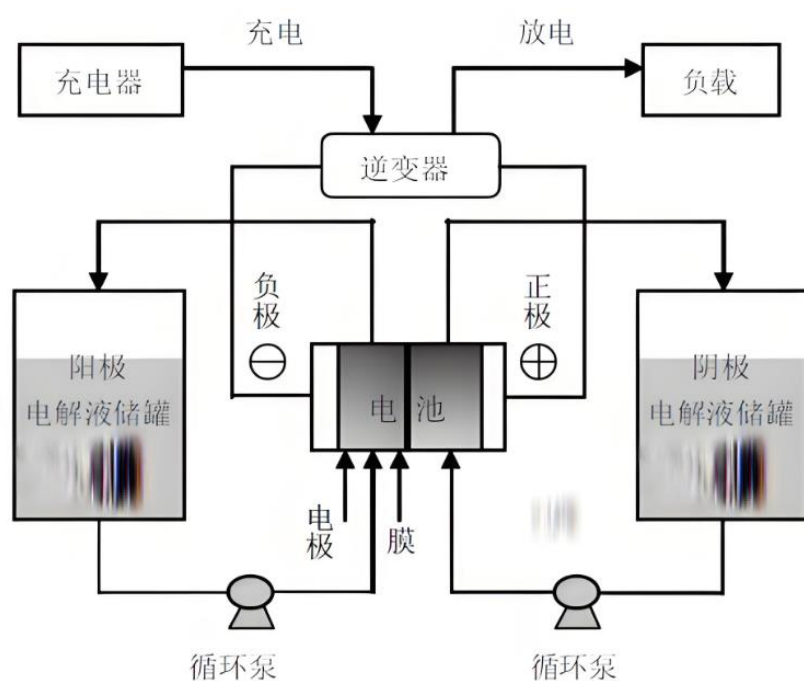
图 11：液流电池工作原理
