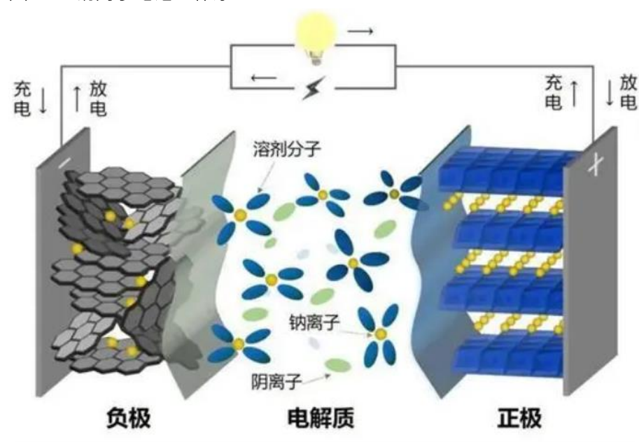
图 10：钠离子电池工作原理
